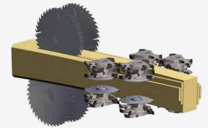
Kantsågen sågar och kantar max fyra optimerade kantbrädor.
