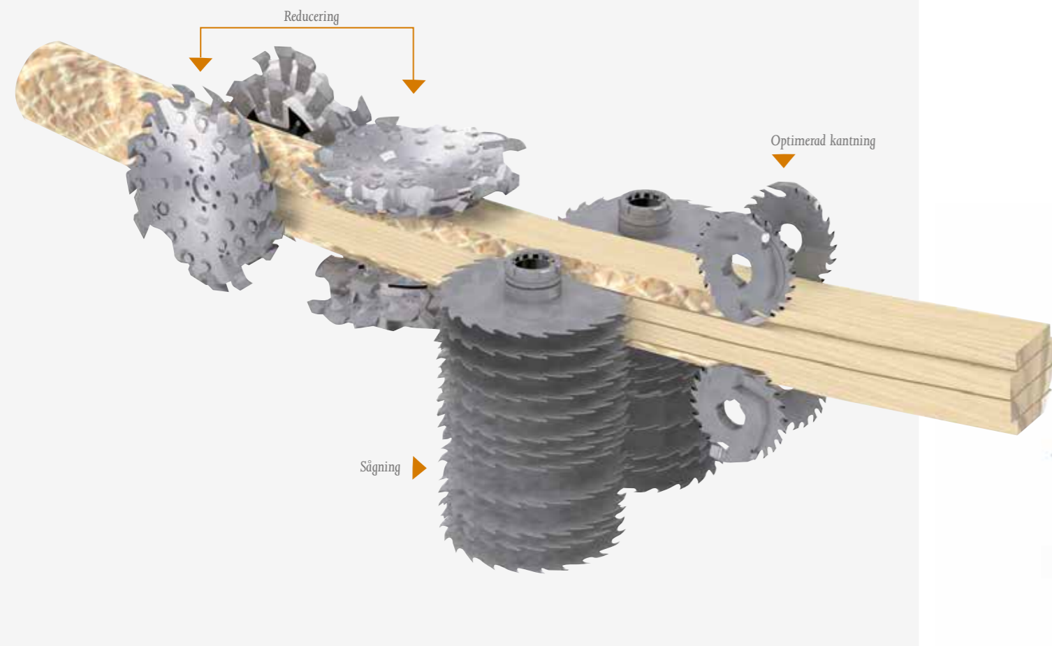
Hög måttnoggrannhet och matningshastighet med HewSaw Log-In
