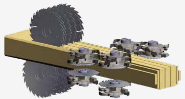
Delningsågen kurvsågar blocket och kantar upp till fyra optimerade kantbrädor.
