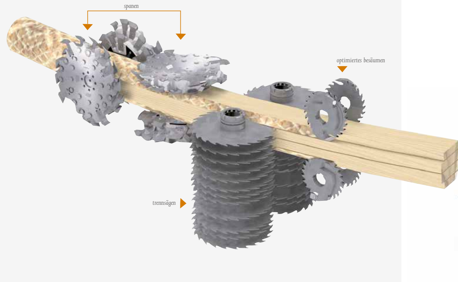
hohe Genauigkeit und Geschwindigkeit mit der HewSaw Log-In
