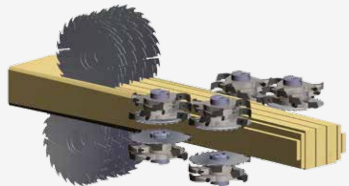
Trennsäge sorgt für den Krumschnitt und besäumt bis zu vier optimierte Seitenbretter
