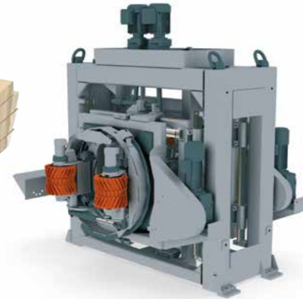
hohe Genauigkeit und Geschwindigkeit mit der HewSaw Log-In
