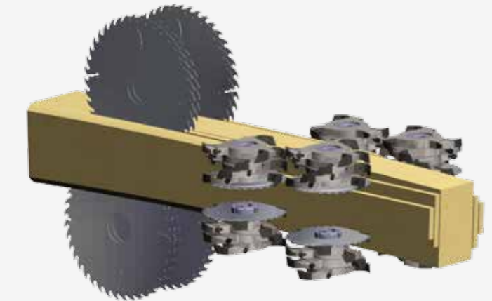
sägt und besäumt das Maximum von vier optimierte Seitenbretter
