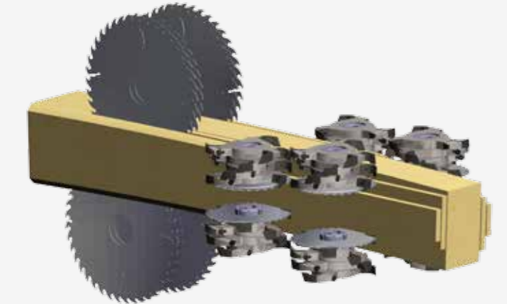
Pelkkasaha sahaa ja särmää optimoidusti neljä sivulautaa.
