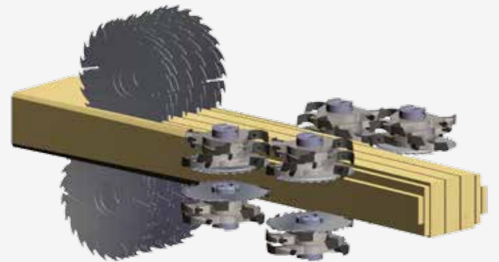
Jakosaha sahaa pelkan ja särmää optimoidusti neljä sivulautaa.
